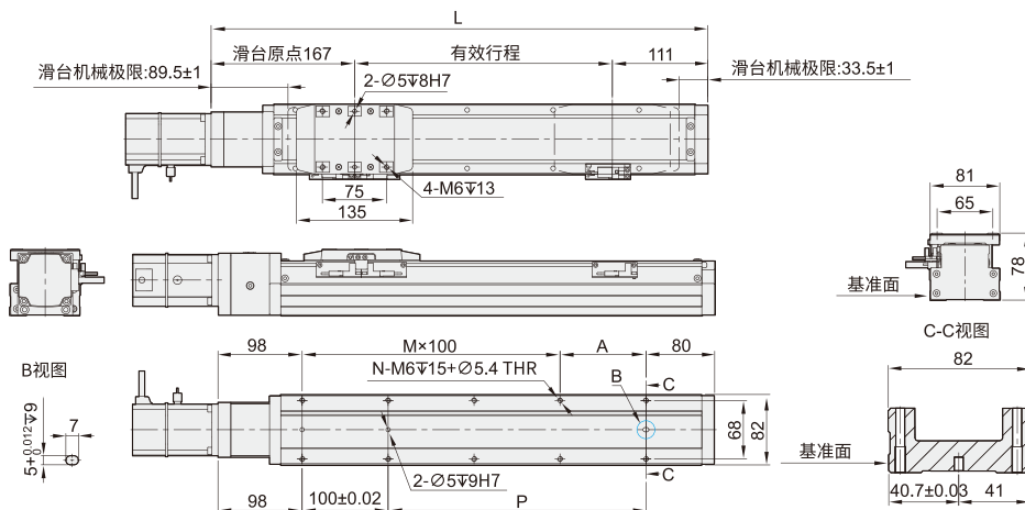
BC马达外露
