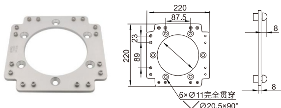
快换连接板
