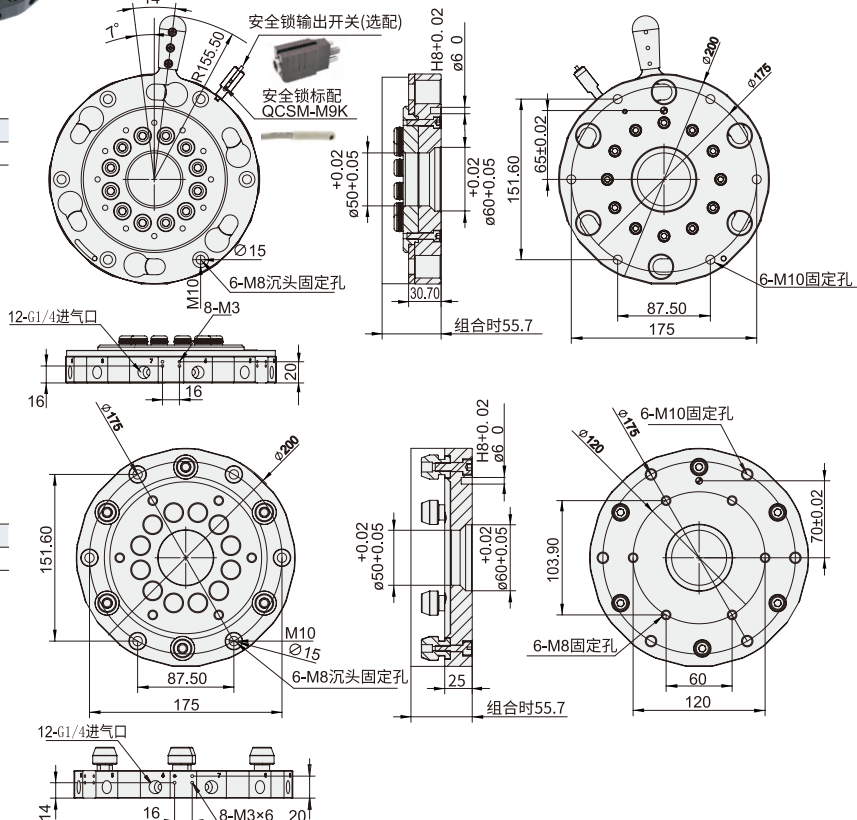
机械手侧的快速转换模块
