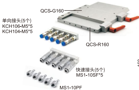
气管接头模组(选配)
