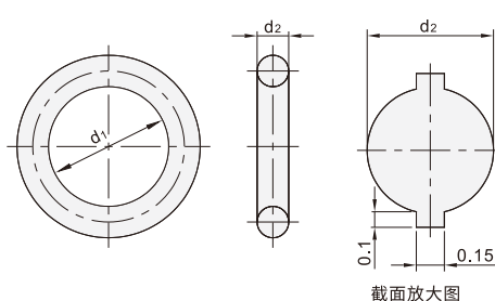
截面放大图
