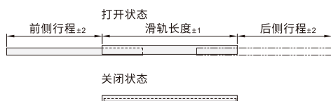
三段式,全长伸展 VZP54
