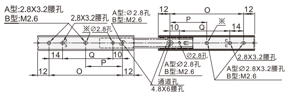
三段式,全长伸展 VZP54
