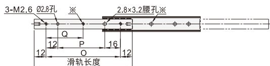
两段式.3/4伸展 VZP53
