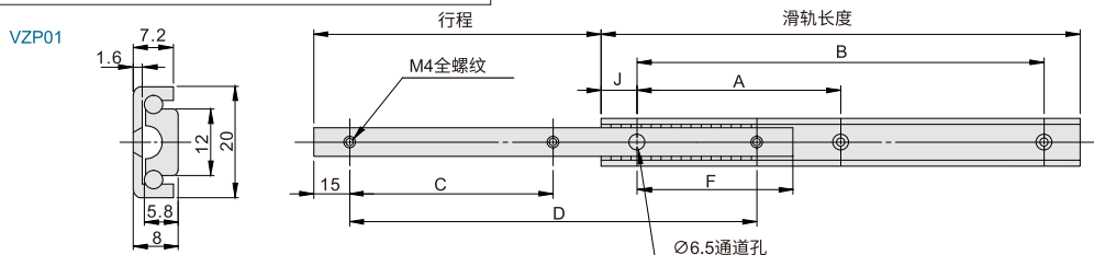
外滑轨安装孔
