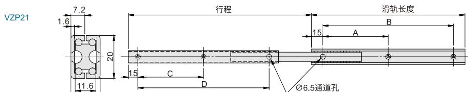
外滑轨安装孔
