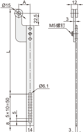
带眼多孔连杆 XAG51
