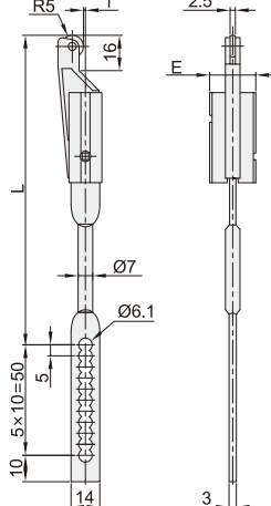
带滚轮连杆 XAG52 XAG53
