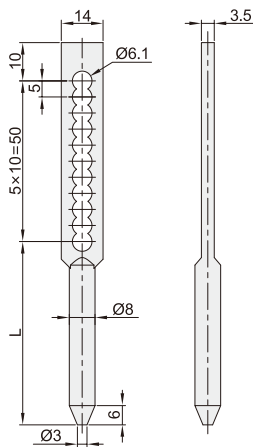
带多孔连杆 XAG41/XAG42
