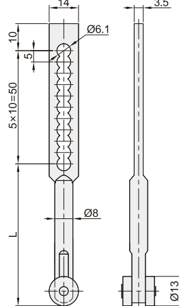
带多孔滚轮连杆 XAG43
