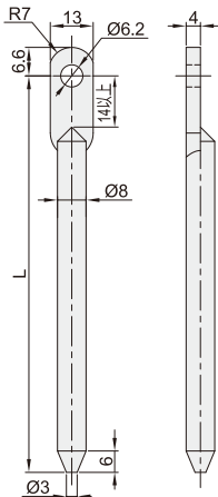
带圆眼连杆 XAG31
