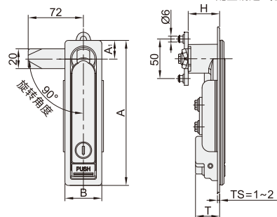
带锁芯 XAD10
