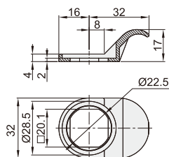
拉手
