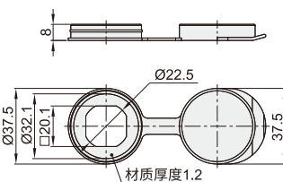
防尘盖
