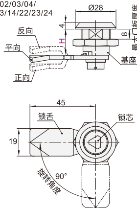
■锁芯形状
