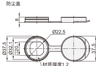
防尘盖
