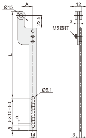
帶眼多孔连杆 CXAG51
