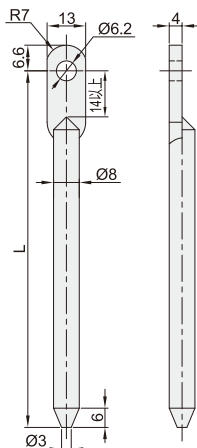
帶圓眼连杆 CXAG31
