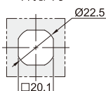
开孔尺寸
