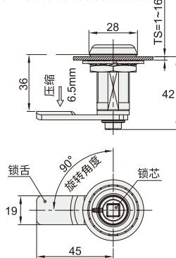
锁芯形状
