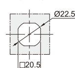
开孔尺寸
