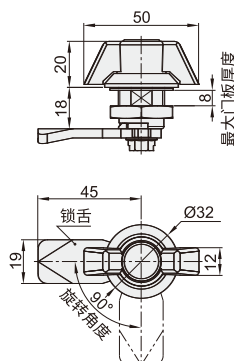
止口高度: 18 无锁芯 XAB49
