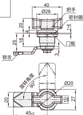
止口高度 25 无锁芯 CXAB47
