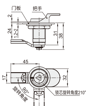
XAB35 止口高度:24
