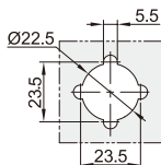
开孔尺寸
