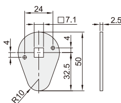
选配件: 三点锁舌
