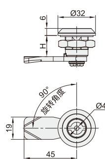
XAB36 XAB37 XAB38 止口高度:30、40
