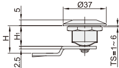
XAB33 止口高度:20 XAB34 止口高度:21
