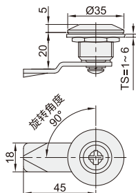
XAB32 止口高度:20
