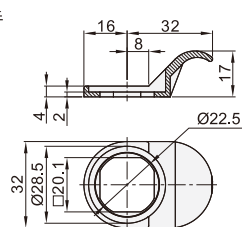
拉手
