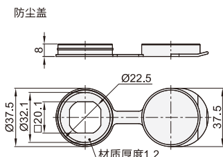
防尘盖
