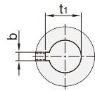
CXL21 键槽圆孔型
