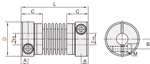
CWA21 螺钉夹紧型
