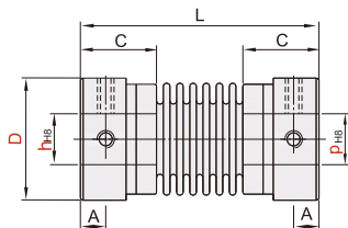
CWA01 螺钉固定型
