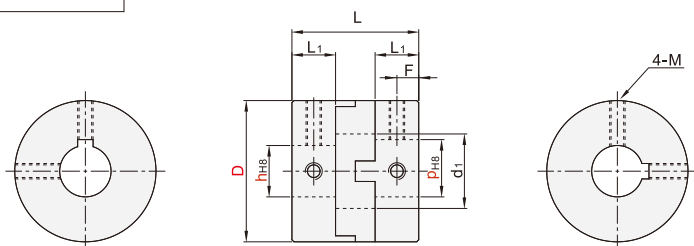
带键槽螺钉固定型 DCHA11
