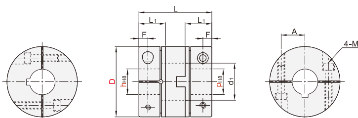
带键槽螺钉夹紧型 DCHA16
