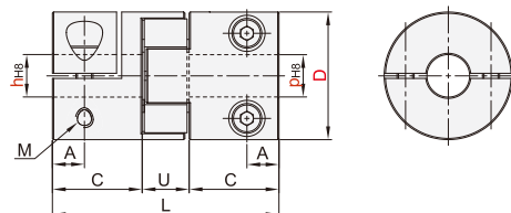
螺钉夹紧分离型 DCEA84
