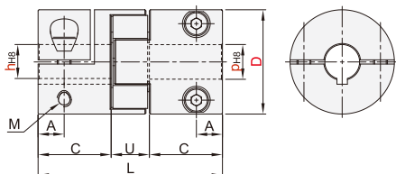
带键槽螺钉夹紧分离型 DCEA83
