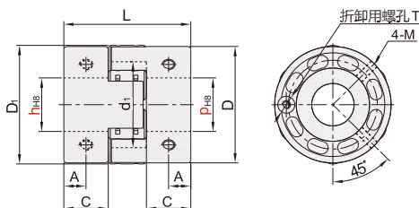
螺钉固定型 CEG02
