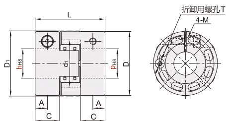
螺钉夹紧型 CEG22
