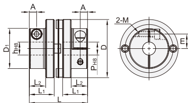
单膜片 CBN01
