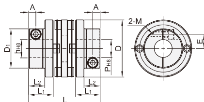
双膜片 CBN21
