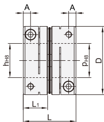
单膜片 CDU01
