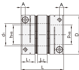
双膜片 CDU11
