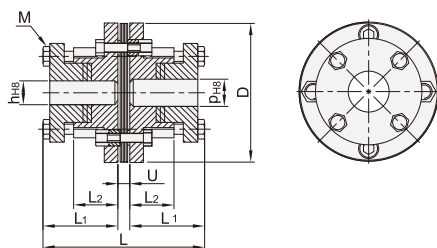
单膜片 CDW01
