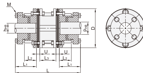
双膜片 CDW11
