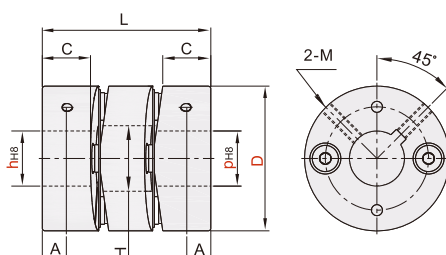
CDR21 螺钉固定键槽型
