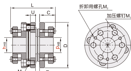
DCDK21 双膜片
