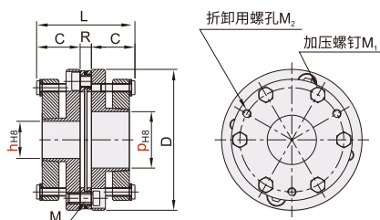
DCDK01 单膜片
