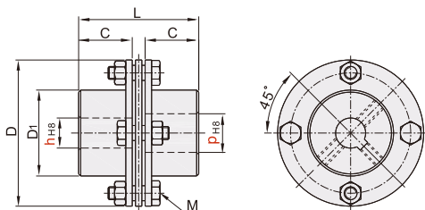
CDJ01 单膜片
