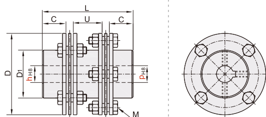
CDJ21 双膜片
