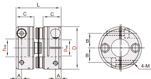
CDB01 单膜片
