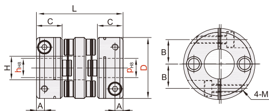
CDB21 双膜片
