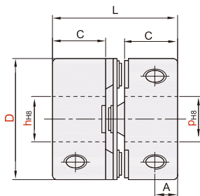
CDH01 单膜片
