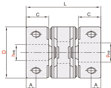
CDH21 双膜片
