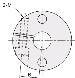
CDG01 单膜片
