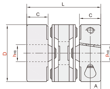
CDG21 双膜片
