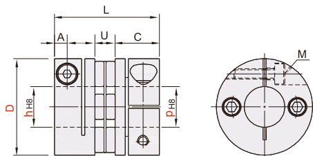
CDE01 单膜片
