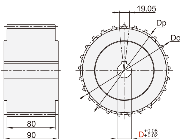
链轮 VXT56
