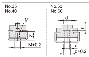
凸型孔加工形状
