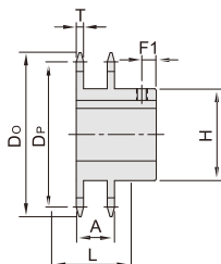
安装方式 (键槽孔型)
