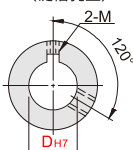
安装方式 (键槽孔型)
