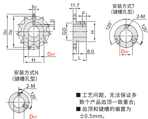
链轮
