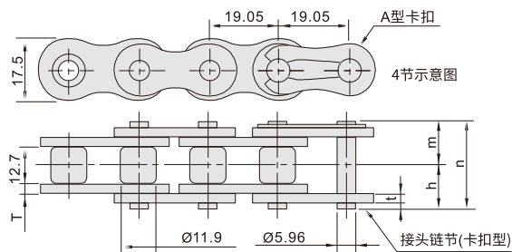
链条
