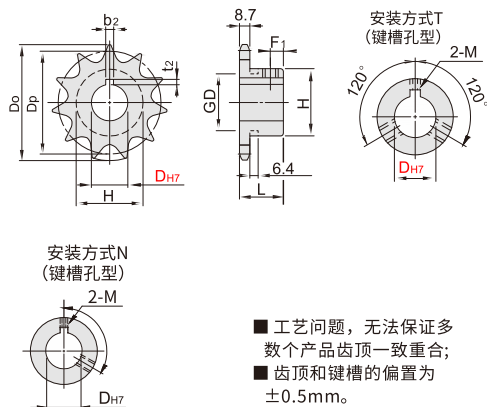
链轮
