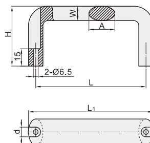
通孔型 VFE06/07
