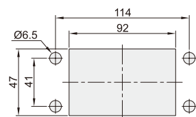
开孔尺寸
