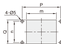
开孔尺寸
