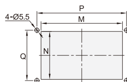
开口尺寸居中
