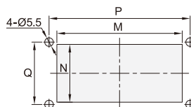
开口尺寸居中
