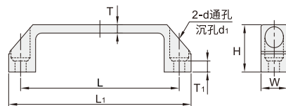
VFT37 VFT38 (L : 100/130) VFT39
