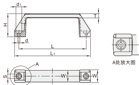
VFT37 VFT38 (L : 100/130) VFT39
