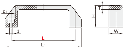
VFT11 VFT12 VFT38 (L : 90)
