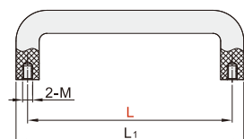
圆角型 VFE21/23
