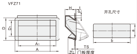
开孔尺寸
