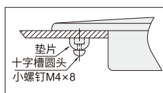
安装图
