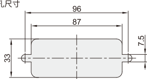
开孔尺寸
