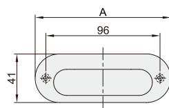
开孔尺寸
