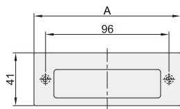
开孔尺寸
