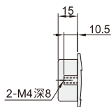
安装图
