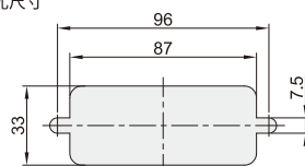
开孔尺寸
