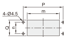
开孔尺寸
