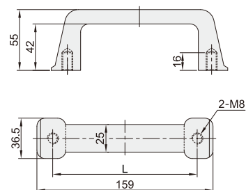
开孔尺寸
