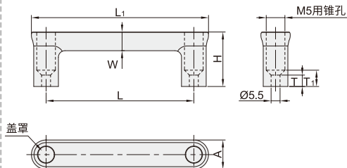
直角带盖型 VFT77/78
