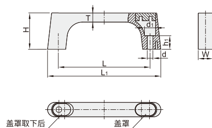
斜角带盖型 VFT76
