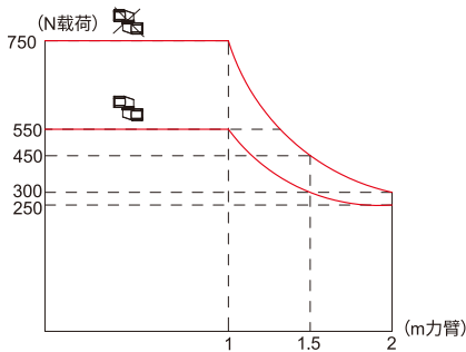
5575系列悬臂组合承重图
