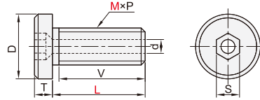
内六角薄圆柱头型 YWK42
