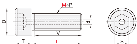
内六角圆柱头型 YWP17
