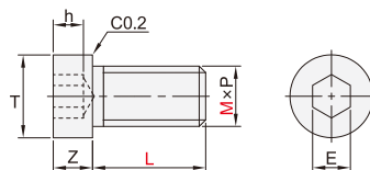
短头小径内六角圆柱头螺钉 YWP13/14
