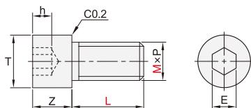
小径内六角圆柱头螺钉 YWP11/12
