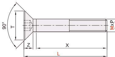
内六角沉头螺钉 YWH01 YWH02
