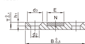
沉头螺栓型 YLG21
