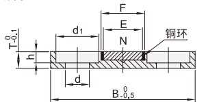
沉孔型 YLG01/06
