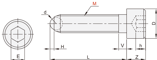
内六角螺栓型 YZL61/62
