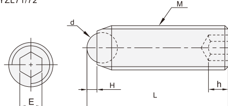
紧定螺钉型 YZL71/72
